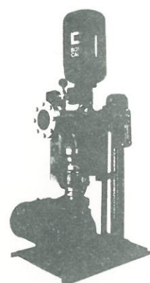
EQUIPOS CONTRA INCENDIOS - Para el abastecimiento de redes contra incendios. Caudal: de 6 m. 3 /h. a 300 m. 3 /h. Presión: de 4 Kg/cm. 2 a 9 Kg/cm. 2 Potencia: de 3 CV a 100 CV. Equipadas con antiarriete de 24 lts. a 200 lts.
